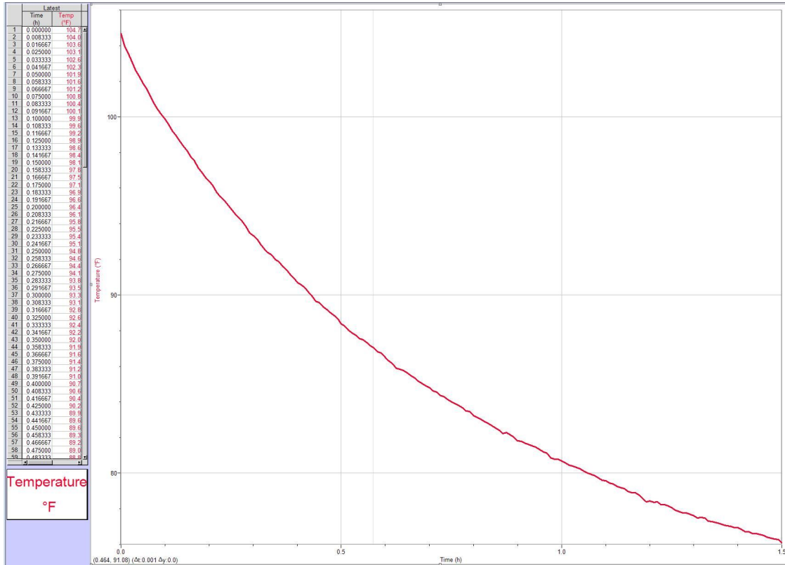
Figura 2. Salida de la pantalla de recopilación de datos de Vernier Software. A la izquierda están las observaciones de tiempo y temperatura con un gráfico a la derecha. En esta situación, la temperatura ambiente o ambiental es 70,3 °F y la temperatura del agua en el vaso de precipitado es inicialmente de 104,7 °F.
